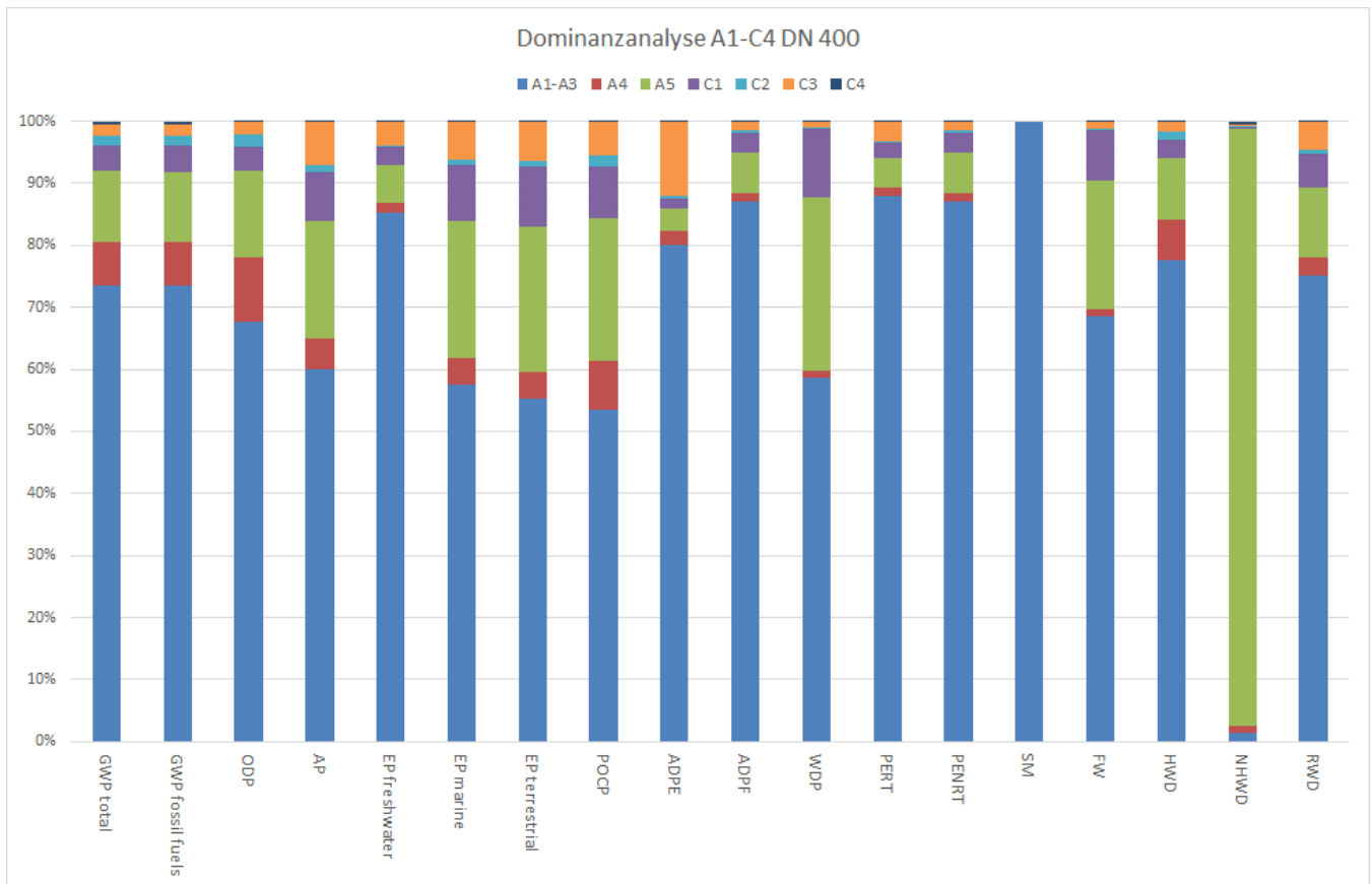
Abbildung 5: Dominanzanalyse DN 400
