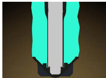
Verpresster Pfahlschuh, Verpresskörper aus Zementmörtel
